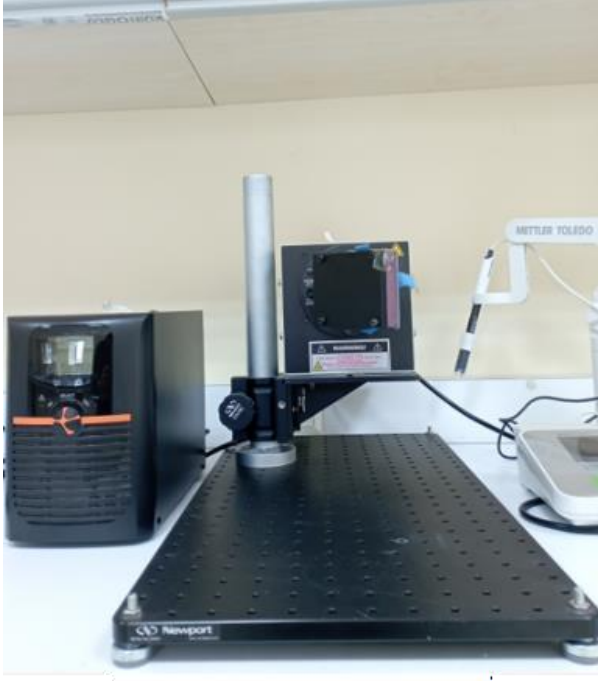
Güneş Simülatörü
